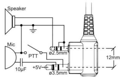
Abbildung 3: Stecker Belegung
